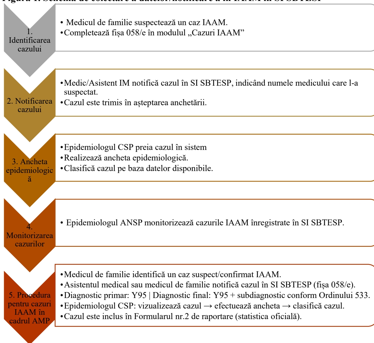
Figura 1. Schema de colectare a datelor/notificare a în IAAM în SI SBTESP
